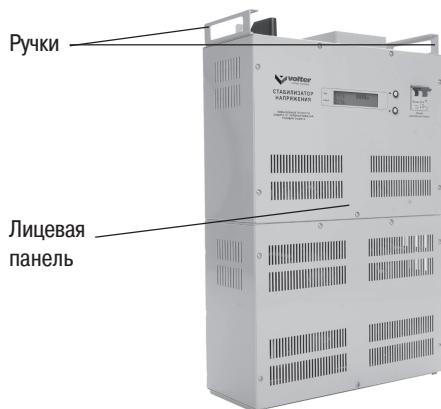
Рис. 1. Стабилизатор напряжения
