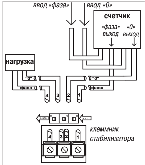
Рис. 17. Схема установки
