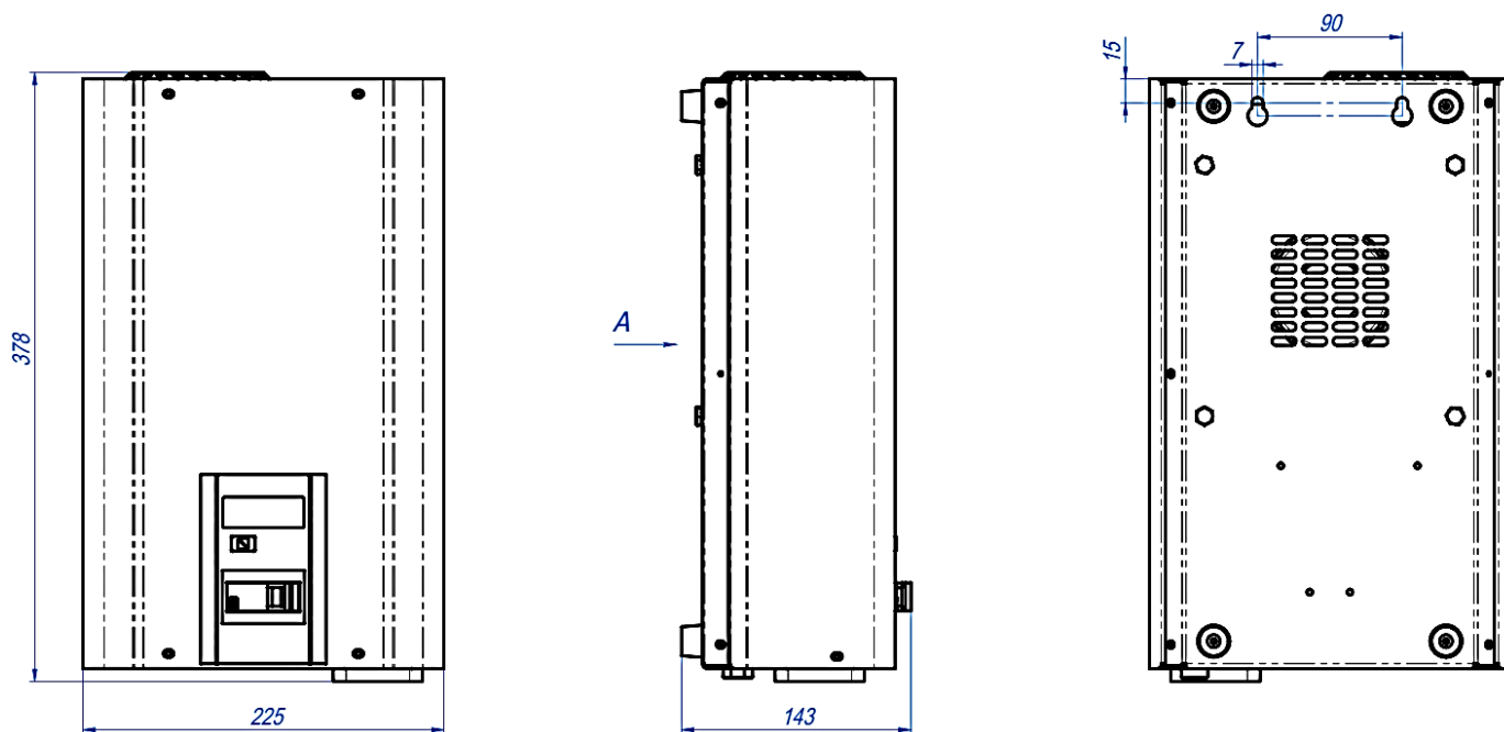
Рисунок 7. Габаритні та установочні розміри стабілізаторів ГБРИД на 10-16А
