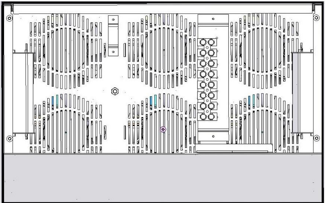
Рисунок 3. Внешний вид верхней части стабилизатора Герц на 25-80А
