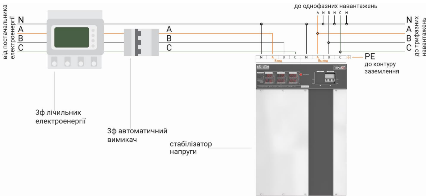
Рисунок 10. Схема підключення стабілізатора до трифазної мережі
